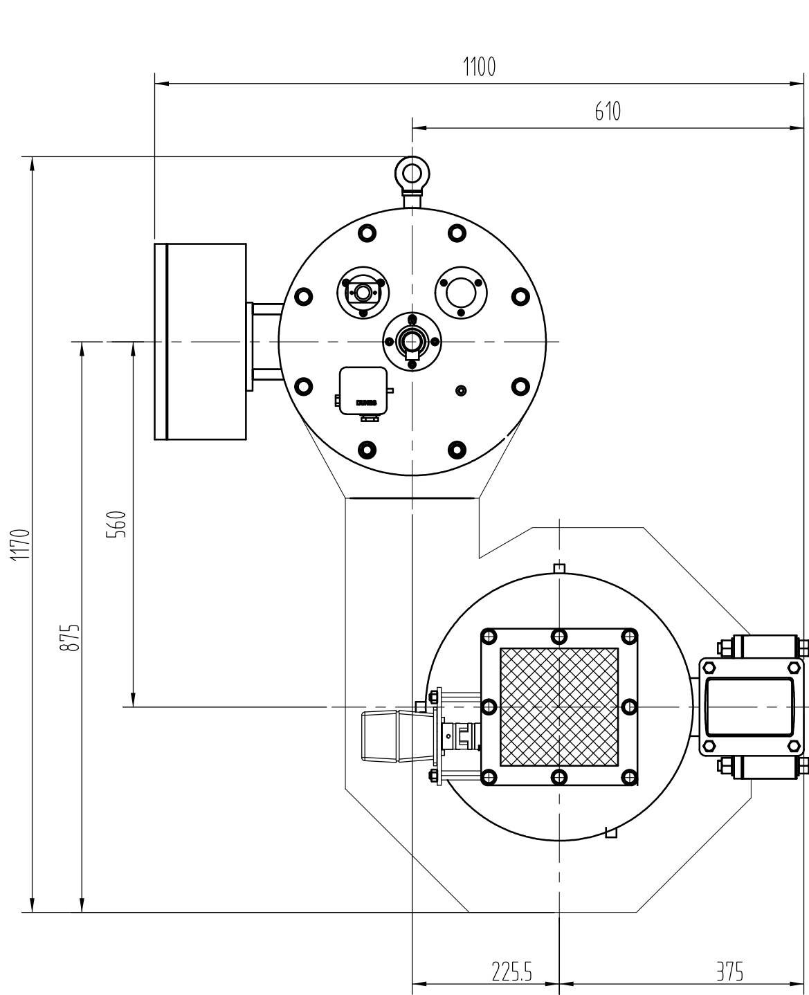
锅炉前板开孔尺寸图
