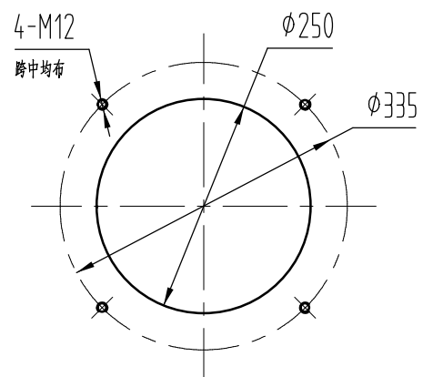
锅炉前板开孔尺寸图
